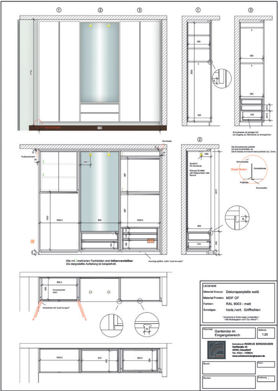
Werkzeichnung
